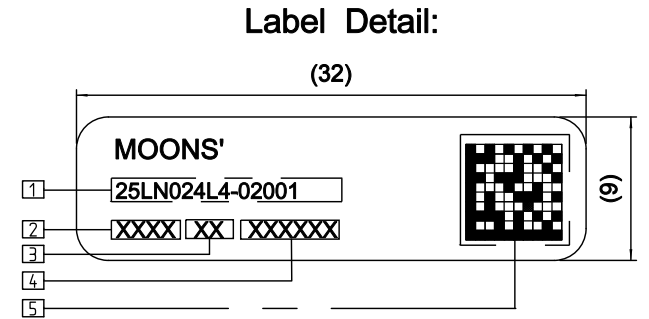
DETAIL A: 2:1
