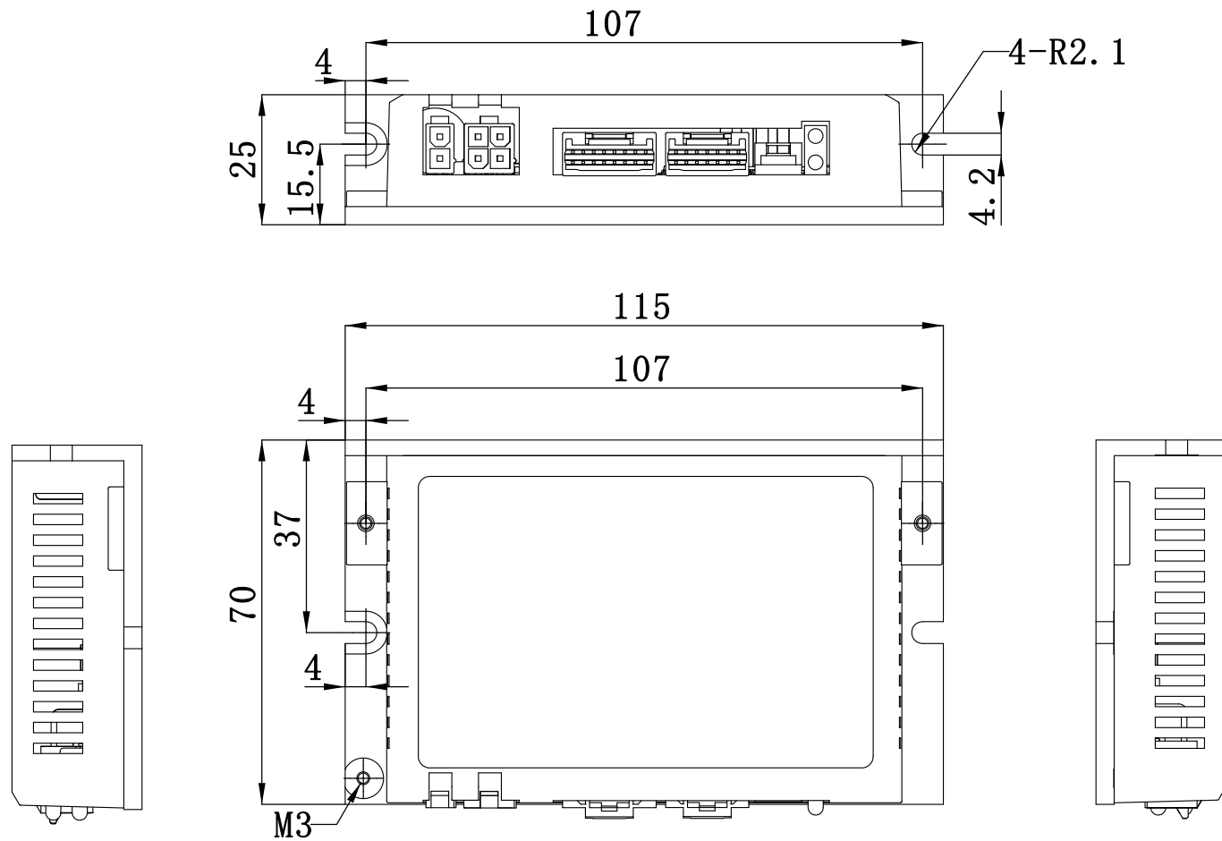
RS-Q/S尺寸图 (RS03-Q-A, RS06-Q-A, RS10-Q-A, RS03-S-A, RS06-S-A, RS10-S-A) RS-Q/S 2D drawing (RS03-Q-A, RS06-Q-A, RS10-Q-A, RS03-S-A, RS06-S-A, RS10-S-A) 比例/Scale 1 : 1 单位/Unit mm 上海安浦鸣志自动化设备有限公司 Shanghai AMP&MOONS' Automation Co.Ltd
